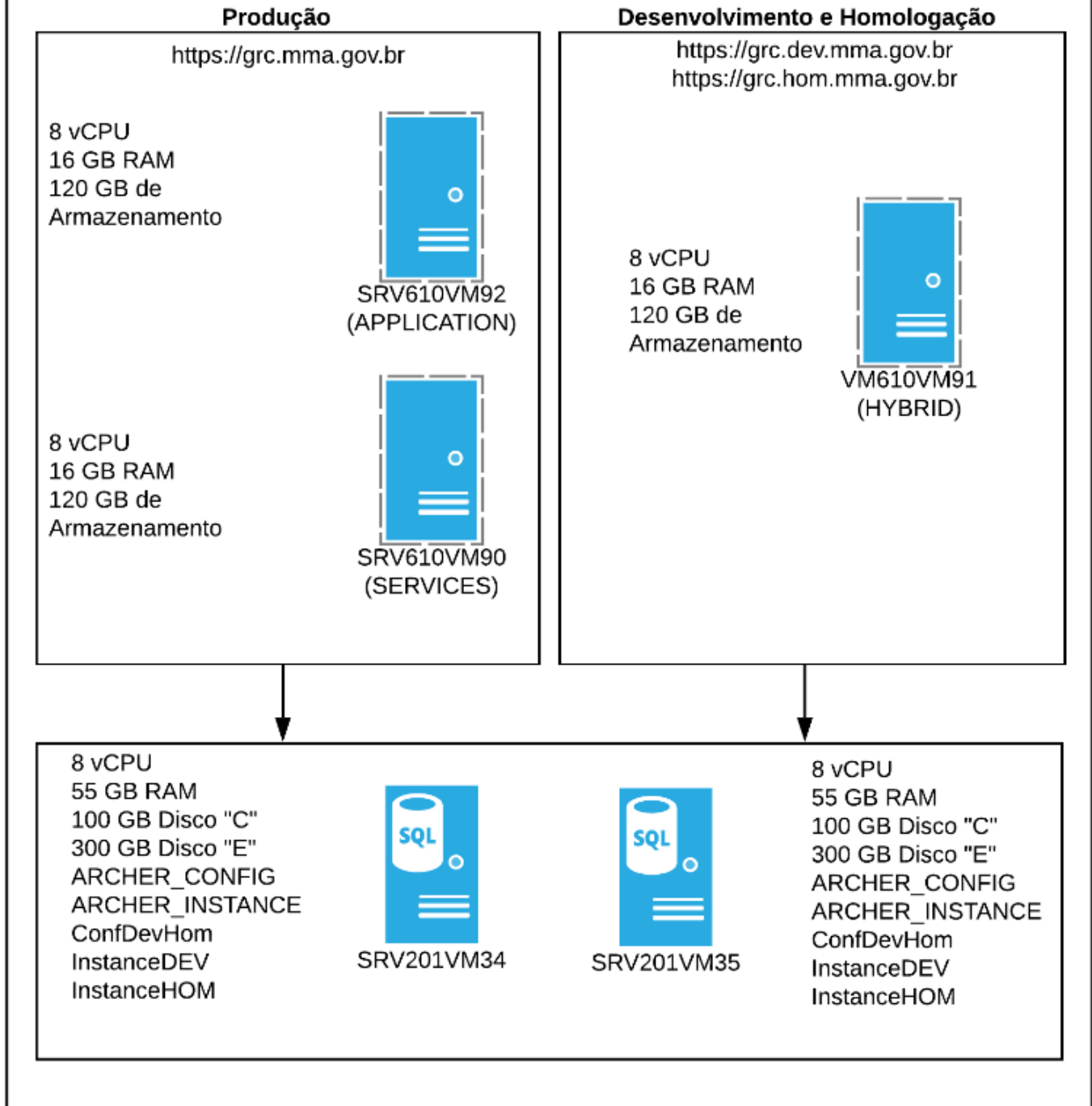
Figura 2 – Topologia da infraestrutura RSA ARCHER SUITE no MMA
