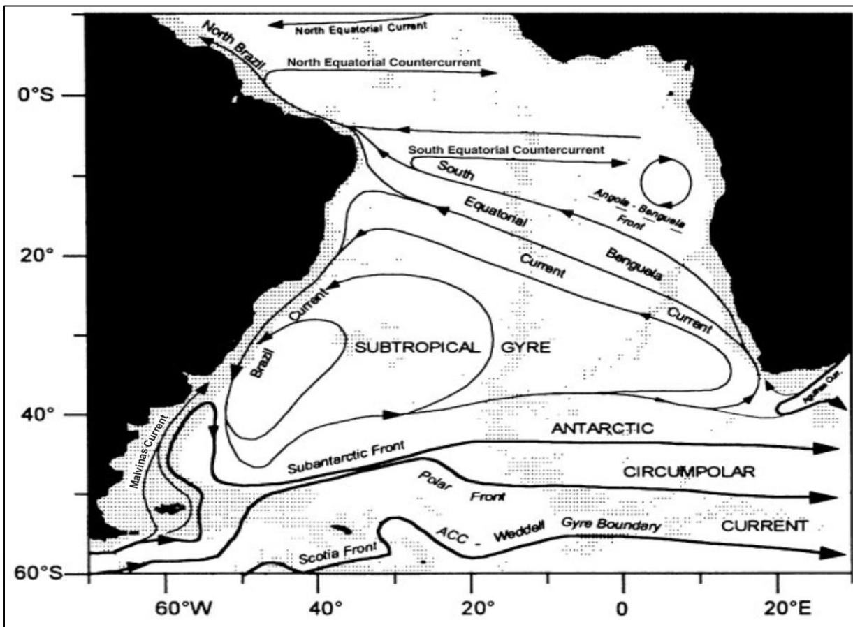
Figura 1. Principais correntes influenciando os processo ecológicos e a biodiversidade no Oceano Atlântico Sul.
