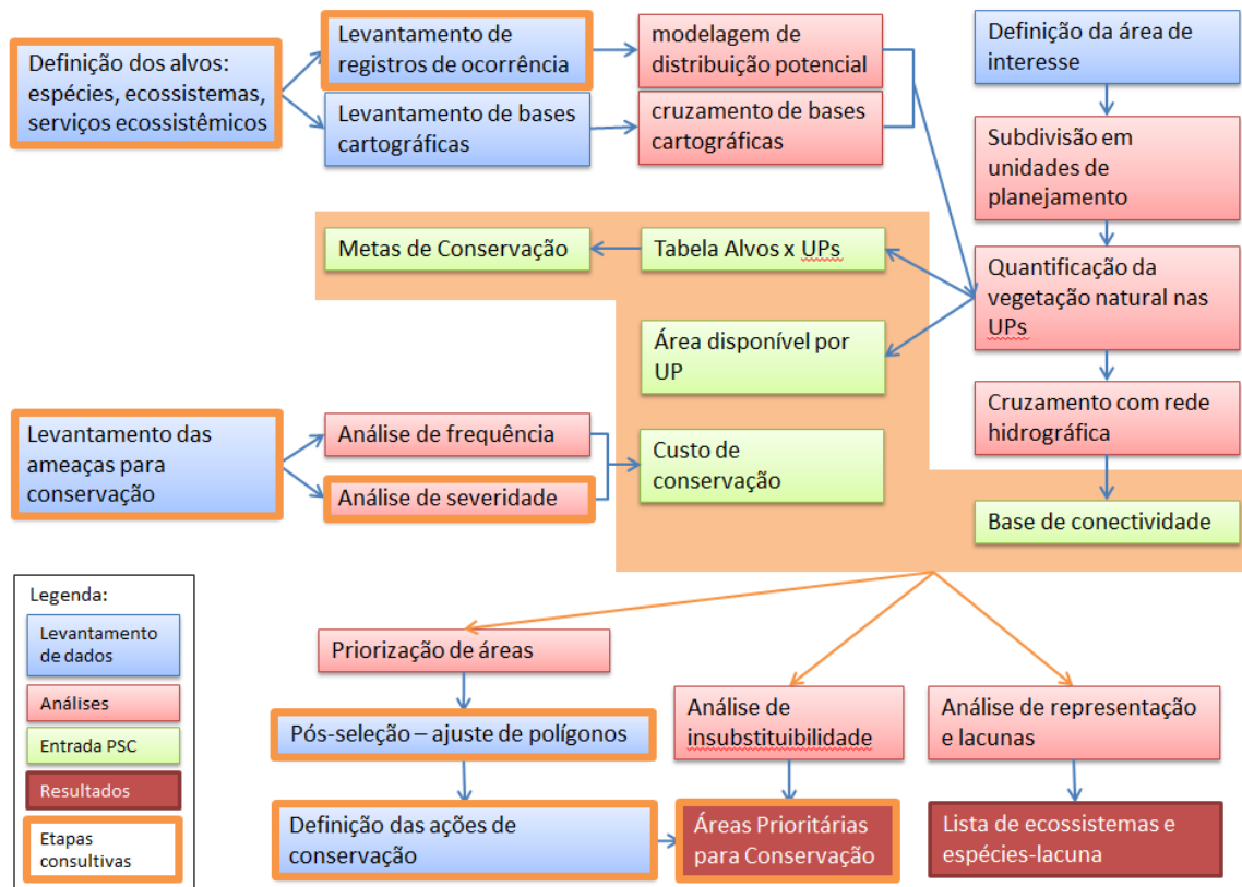
Figura 1: Fluxograma descrevendo as etapas do processo de análise de representação ecológica e identificação de áreas complementares ao sistema de unidades de conservação.
