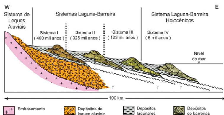
Figura 4 - Corte esquemático mostrando a estrutura da Planície Costeira do Rio Grande do Sul (Modificado de Tomazelli & Villwock, 2005). Fonte: Lopes et al. (2008).
